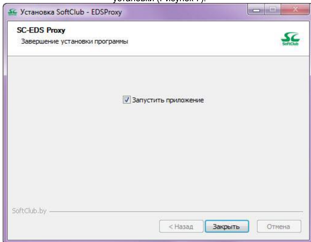
Рисунок 7 – Завершение установки
