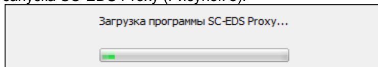
Рисунок 8 – Процесс запуска
