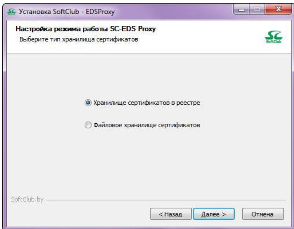
Рисунок 4 – Тип хранилища
