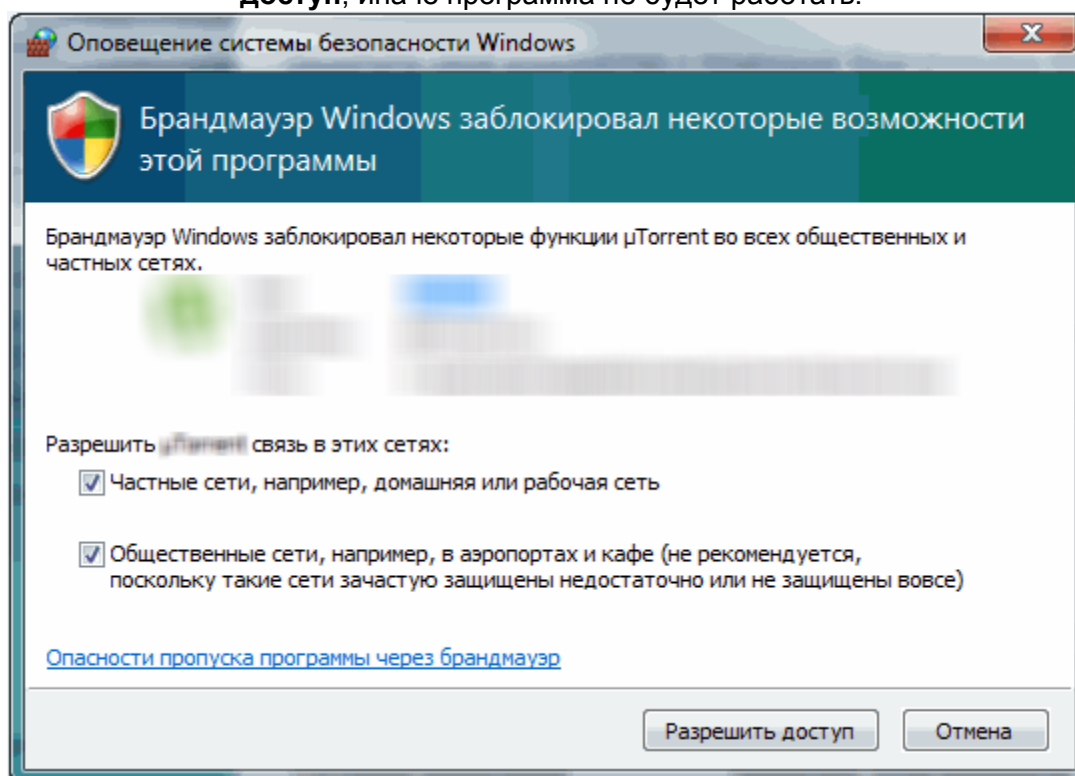
Рисунок 9 – Брандмауэр Windows
